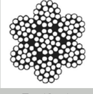
7 x 19 wire
